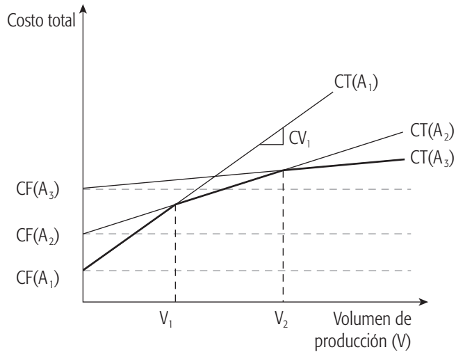
Gráfico 7.7 Funciones lineales de costo total de alternativas tecnológicas
