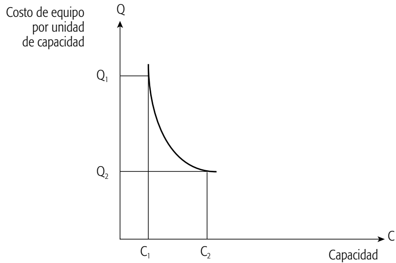
Gráfico 7.2 Costo distribuido de los equipos por unidad de capacidad
